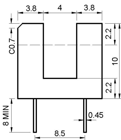
主视图
