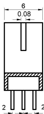
剖视图
