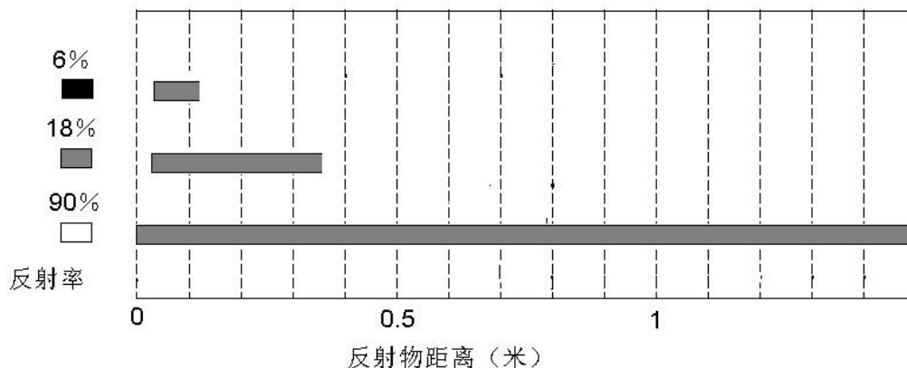
反射率与检测距离关系示意图
