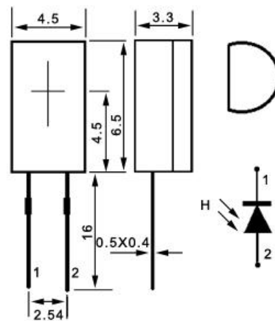
外形尺寸 (mm) 及内部电路图
